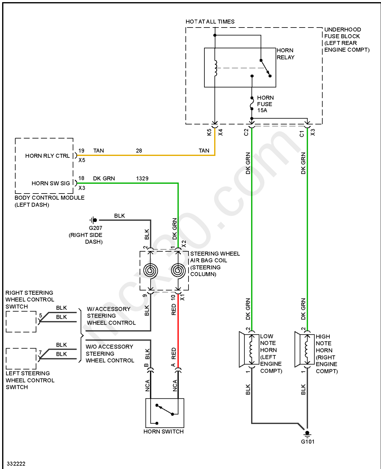
Fig. 37: Horn Circuit
