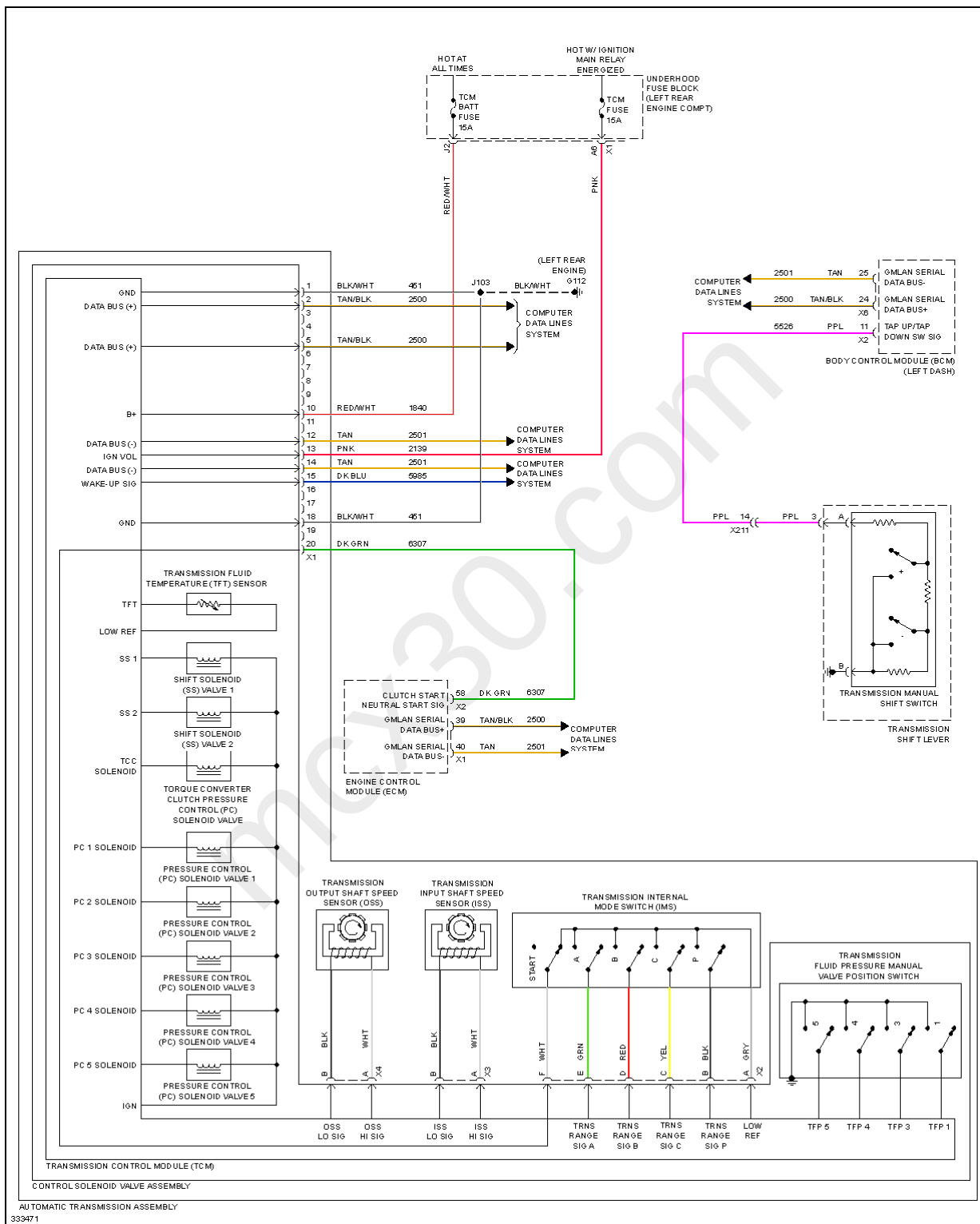
Fig. 77: 3.0L VIN Y, A/T Circuit
