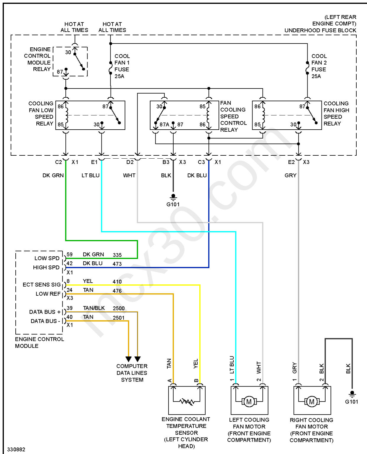
Fig. 15: 3.0L VIN Y, Cooling Fan Circuit
