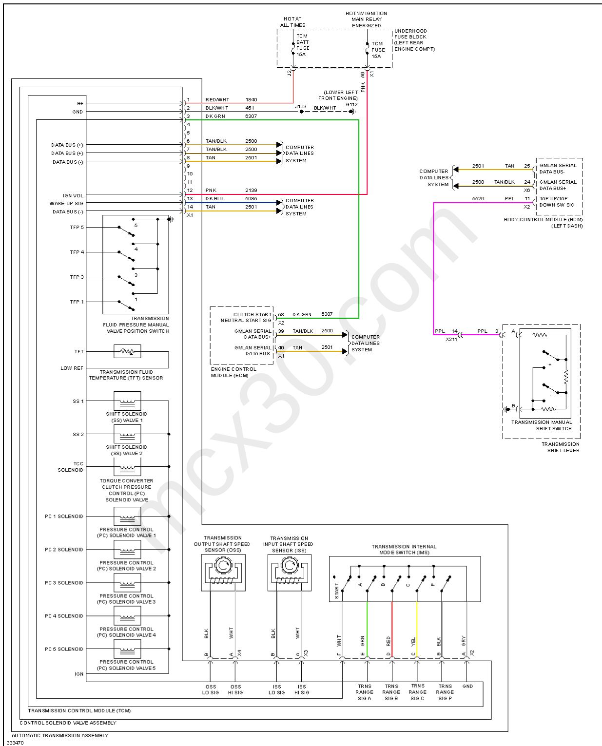
Fig. 75: 2.4L VIN W, A/T Circuit
