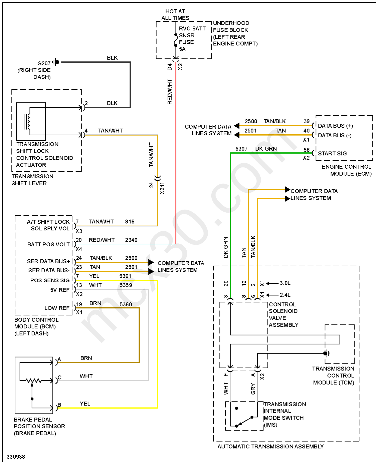
Fig. 70: Shift Interlock Circuit
